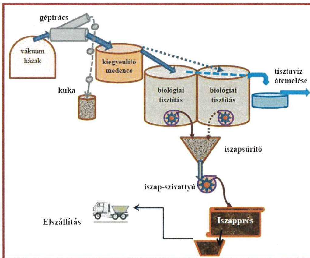
Szennyvíztisztítási technológia folyamatábrája
